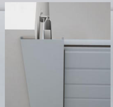
Montage in der Öffnung - Abdeckungen vor der Öffnung
