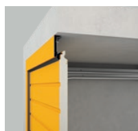
Montage in der Öffnung – Abdeckung in der Öffnung
