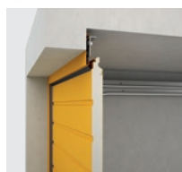
Montage hinter der Öffnung – Abdeckung hinter der Öffnung
