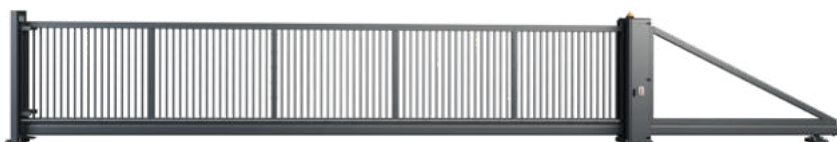
Profilfüllung 30x18 [mm] (in der Konstruktion angeschweißt)
