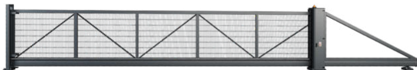
Füllung mit Gitterpaneelen VEGA 2D Super (angeschraubt)
