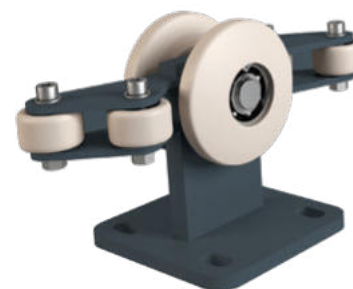
Laufwagen bei PI 130-Toren
