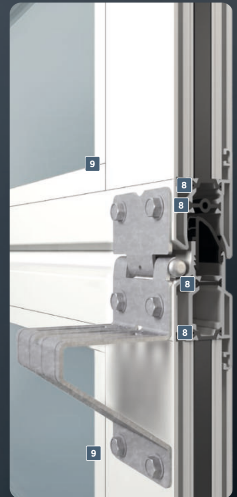
Verglasung für Tore MakroPro 2.0, MakroPro 100 2.0
