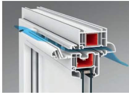
Hyrogesteuerter Lüfter Aereco EMM
