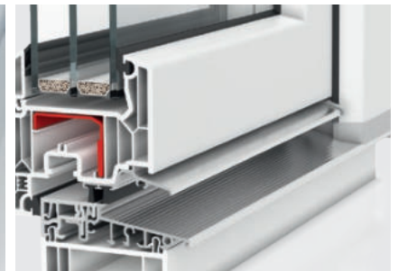
Niedrige Aluminiumschwelle
