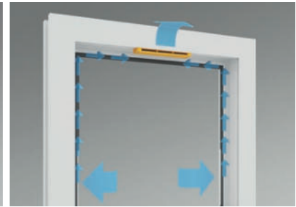
Verdeckter Falz-Lüfter MACO Vent
