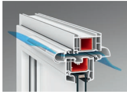
Drucklüfter Aereco AMO
